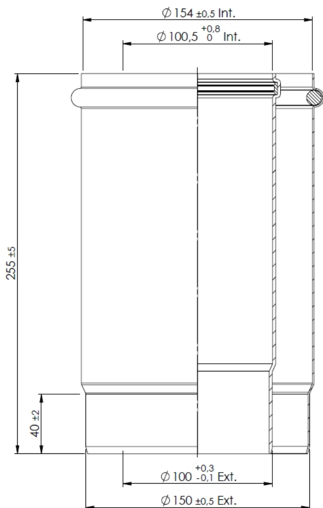
SECTION A-A
