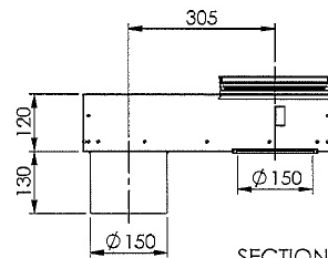
SECTION A-A SCALE 1 : 10
