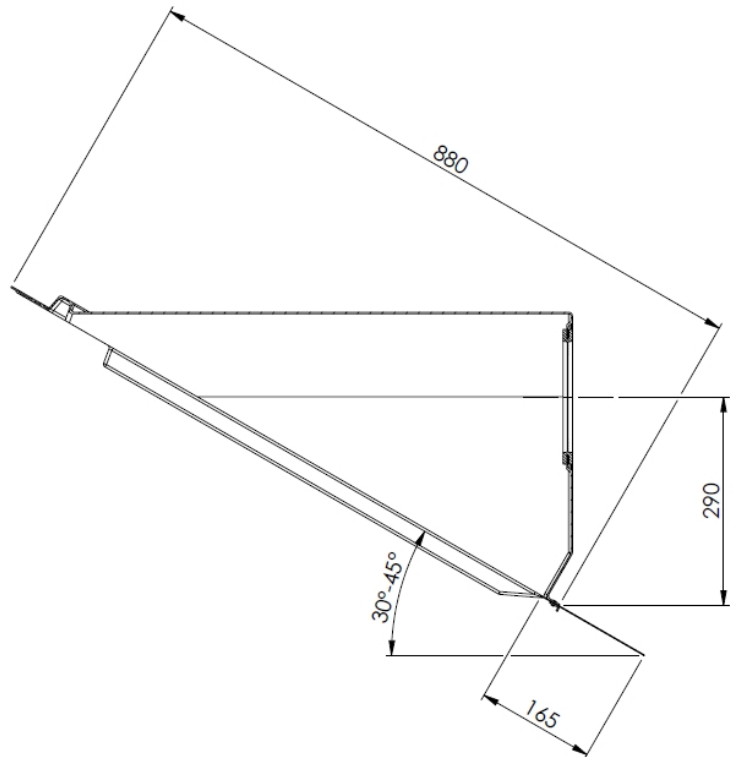
SECTION A-A
