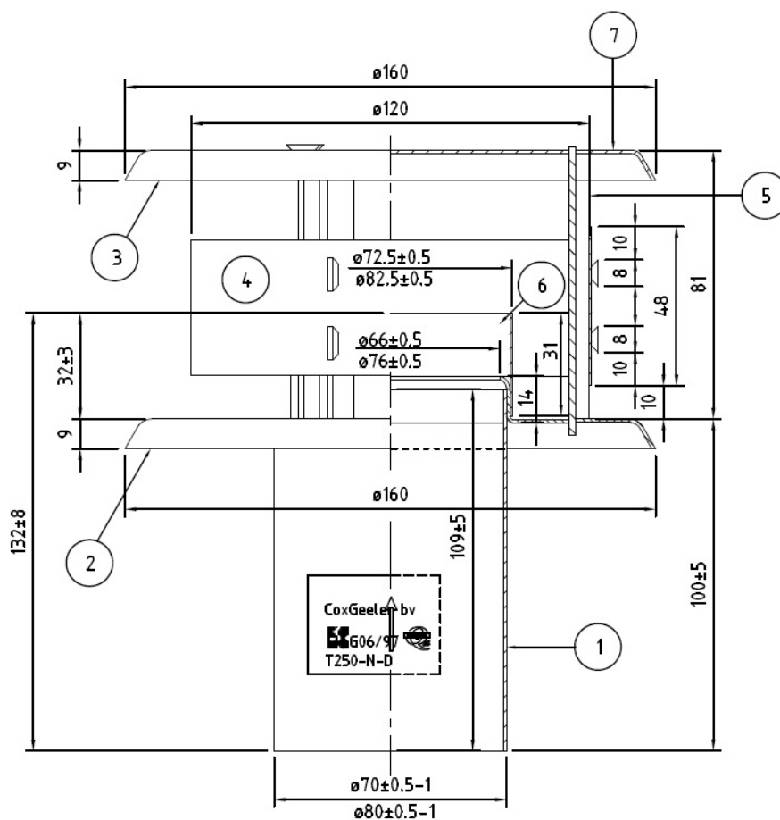
DSN A-A
