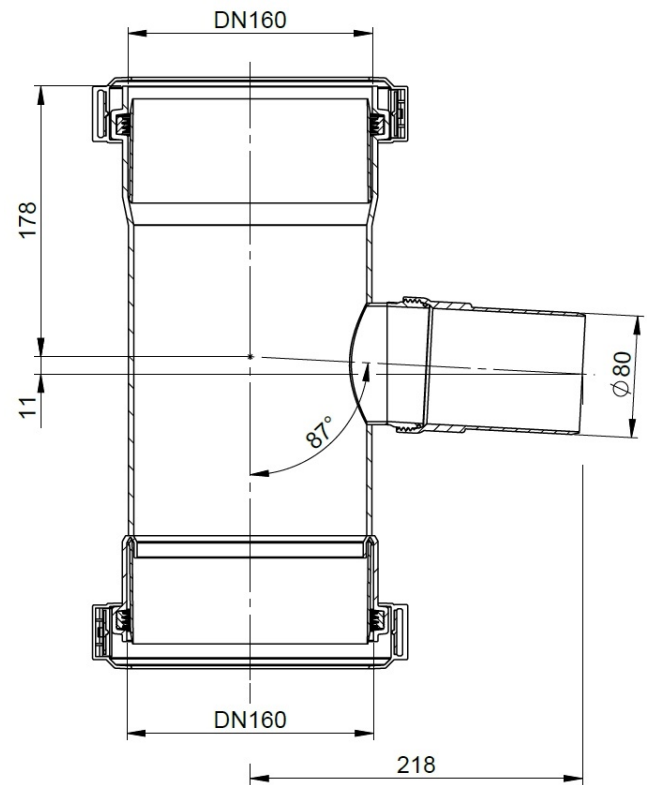
B-B
