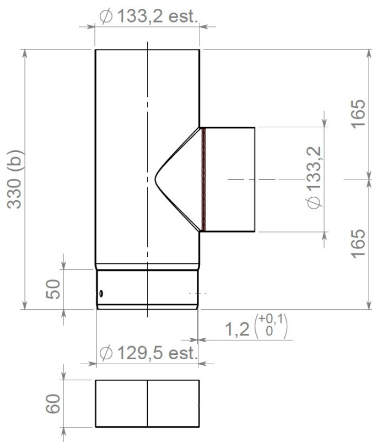
Sectie A-A
