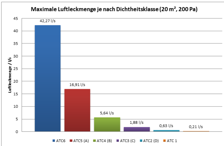
Fig 44 : Graphique du débit maximale selon la table 3
