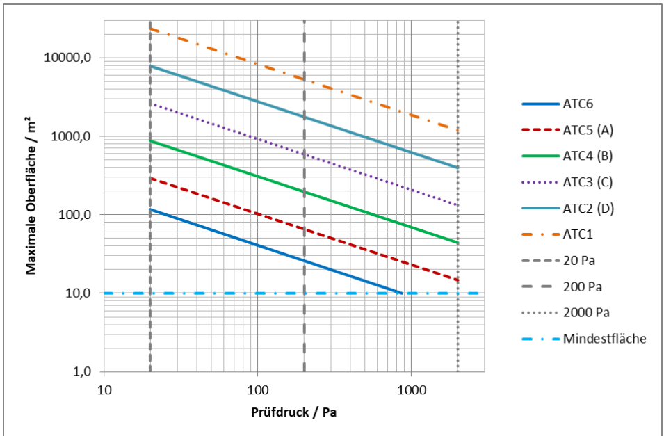
Fig. 43: Grafique: Pression de test en fonction de la surface selon la classe d'étanchéité A - D
