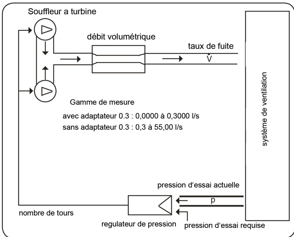
Fig. 9 : Principe de mesure, test d'étanchéité avec le Wöhler DP 700
