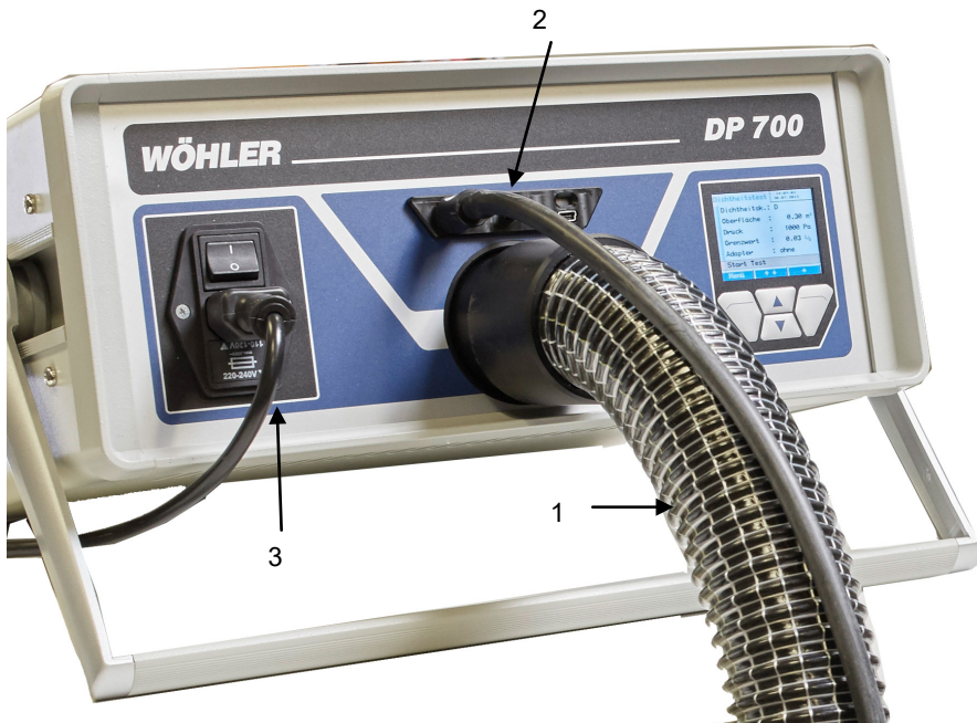
Fig. 2: Raccords des flexibles sans adaptateur
