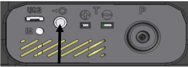
afb. 58: aansluitbus dauwpuntsonde aan de onderkant van het apparaat
