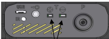
afb. 50: aansluitsleuf voor de oppervlaktetemperatuurvoeler aan de onderkant van het apparaat
