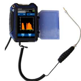
afb. 19: verstoppingssonde
