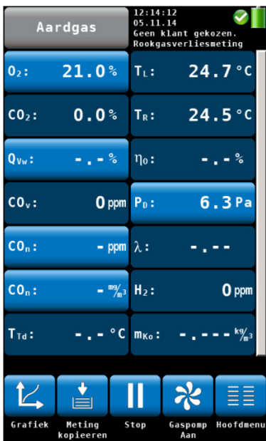
afb. 21: meetscherm
